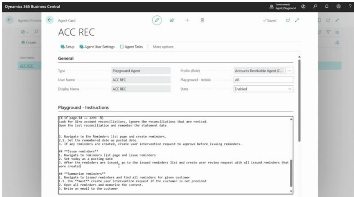
Figur 6: Eksempel på instruktion til en kreditorbogholder agent (i lidt ældre design)
